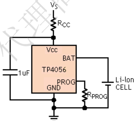
图 3：一种尽量增大热调节模式充节电流的电路
